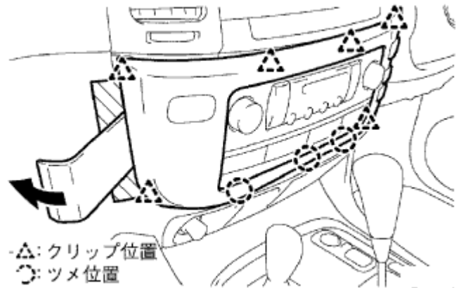
デッキ周辺パネルを外します
