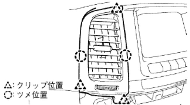
パネルを外します 右側も同様
