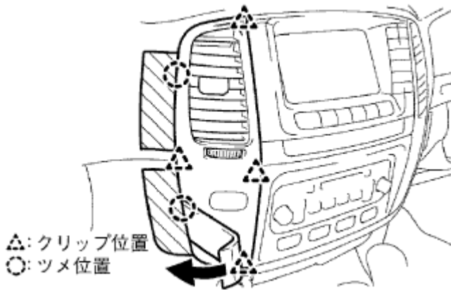
パネルを外します 右側も同様
